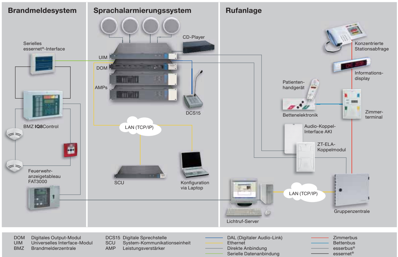
Prinzipschaltung für die Anbindung von Sprachalarmierungskomponenten an die Gewerke Brandmeldetechnik und Pflegekommunikation
